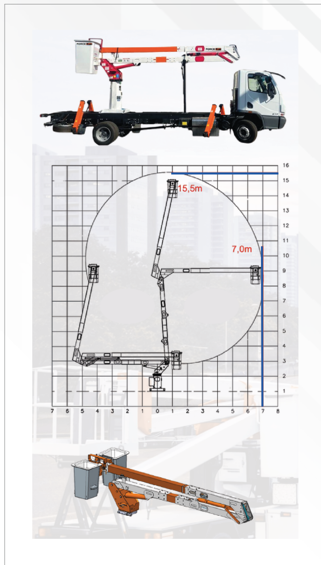
DIAGRAMA DE CARGA
